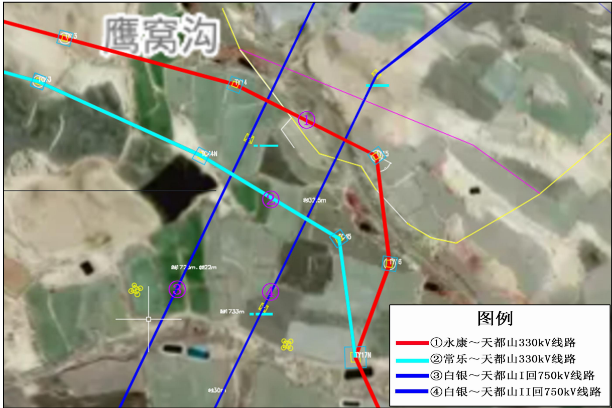
图 6.1-14 本项目交叉钻越线路示意图（2）
