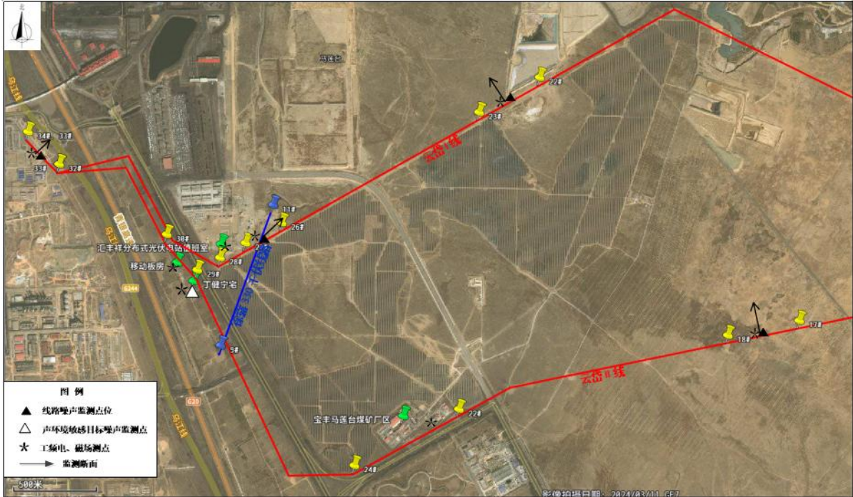
图 6.1-2 类比 330 千伏云岱I线单回路、云岱I、II线同塔双回路段监测点位示意图
